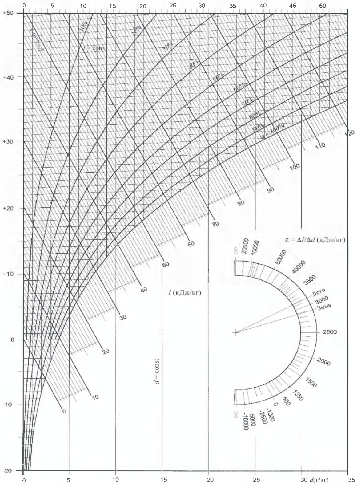
J – d диаграмма влажного воздуха
