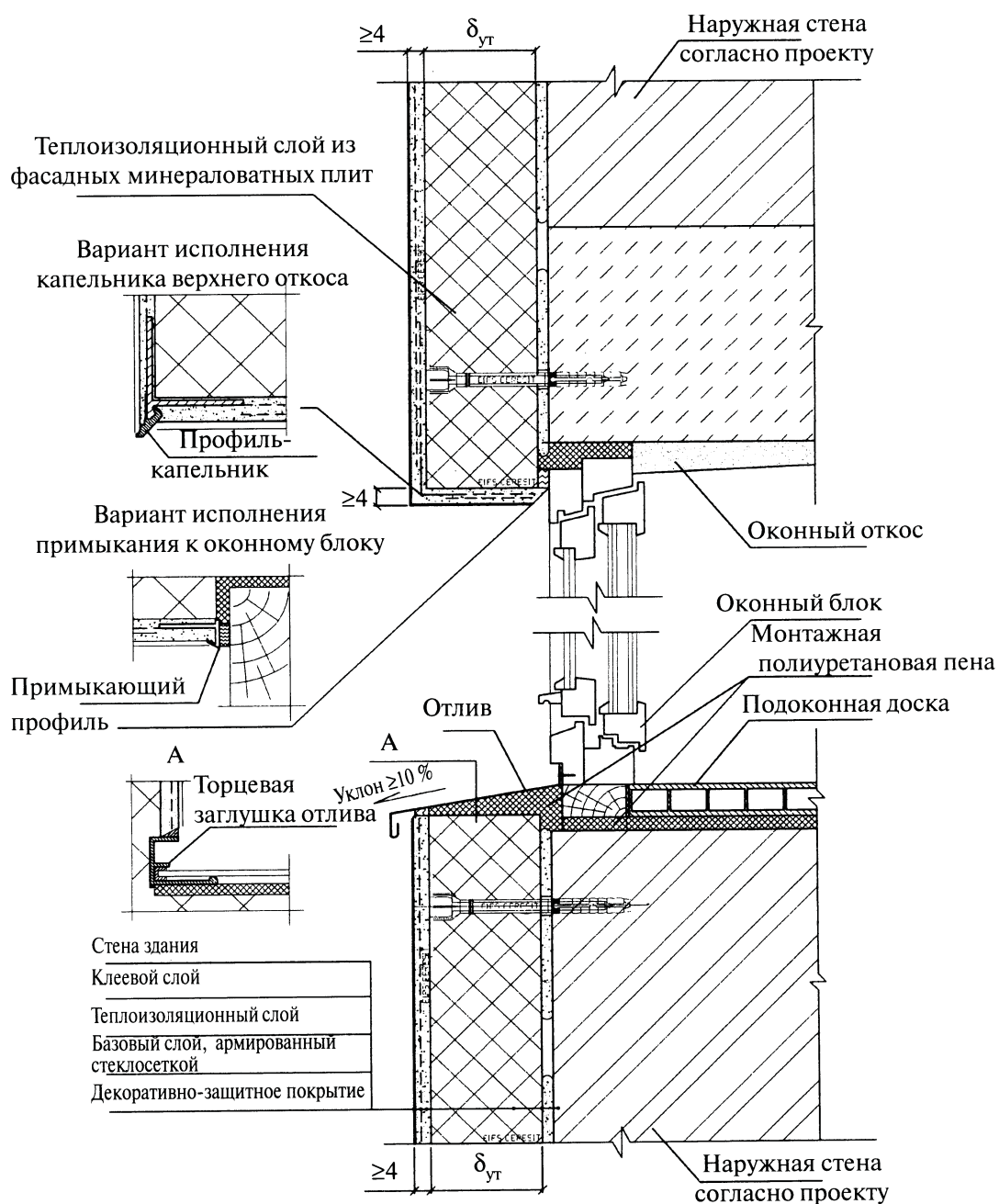
Рисунок 5 – Узел примыкания СФТК к оконному блоку (пример)
